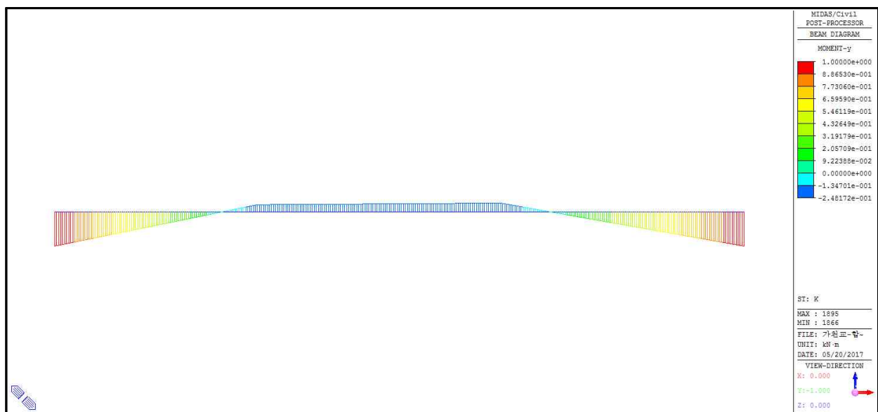
<그림 5.2.3> 부정정력에 의한 영향을 고려하기 위한 K값 산정
