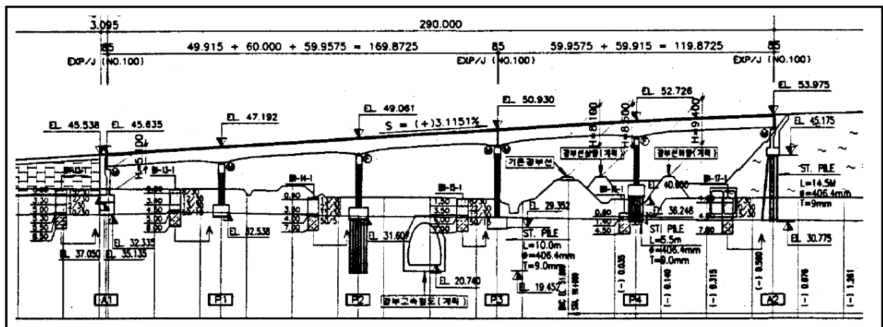
a) 종단면도
